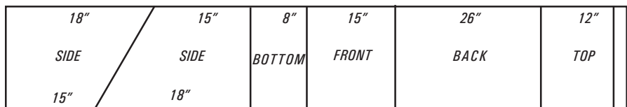
Plank 1” x 10” x 8’ cut diagram
